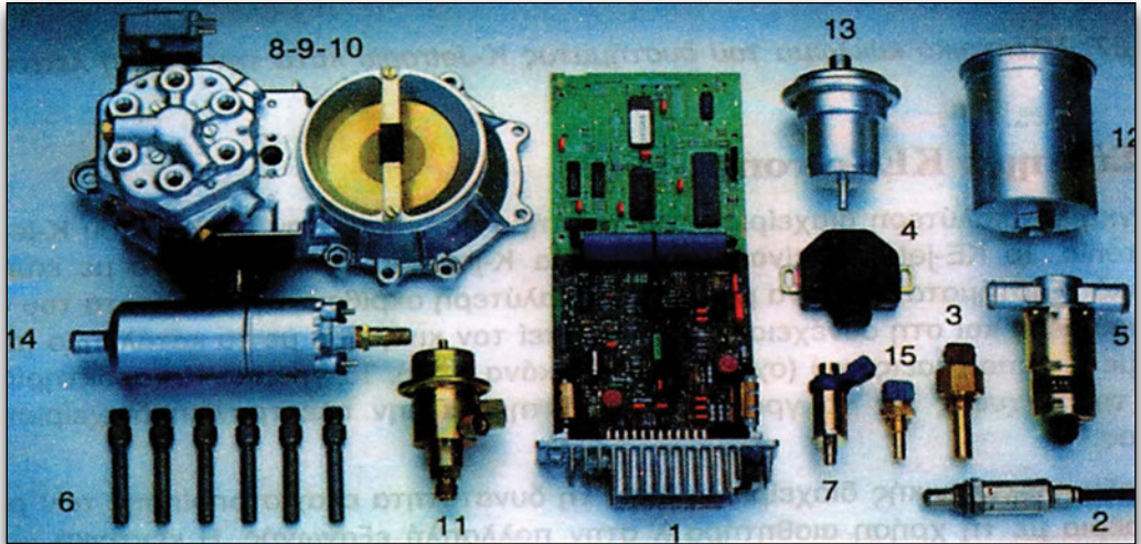
Εικόνα 3.1.47 Εξαρτήματα ΚΕ –Jetronic
