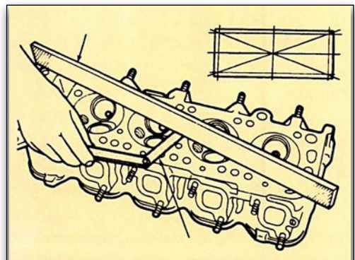
Εικόνα 2.1.3 Έλεγχος επιπεδότητας
