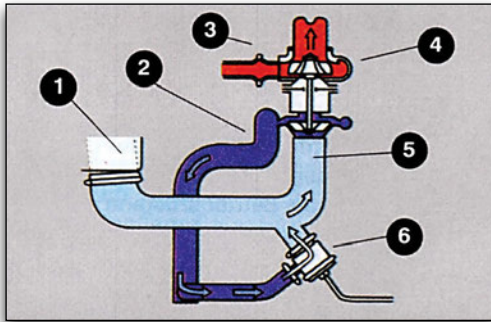
Εικόνα 2.5.11 Σύστημα με βαλβίδα ανακύκλωσης
