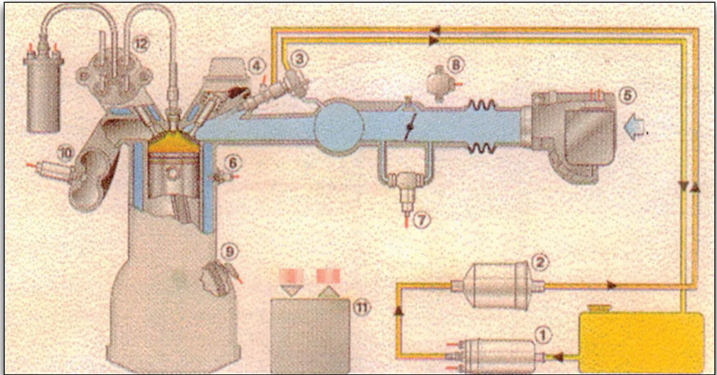
Εικόνα 3.3.4 Εξαρτήματα Motronic
