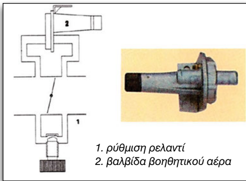
Εικόνα 3.1.39 Μπάι-πας και βαλβίδα βοηθητικού αέρα (τσοκ)
