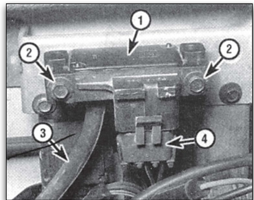
Εικόνα 3.1.30 Αισθητήρας υποπίεσης πολλαπλής εισαγωγής (MAP)
