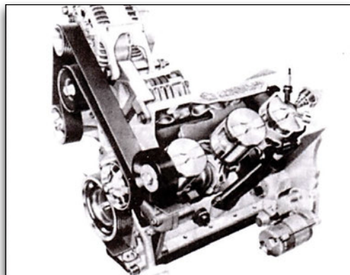
Εικόνα 1.2.8 Δίχρονος βενζινοκινητήρας
