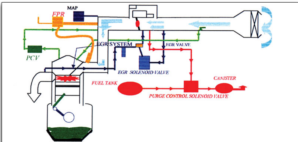
Εικόνα 4.1.1 Συνδεσμολογία και συστήματα ελέγχου ρύπων
