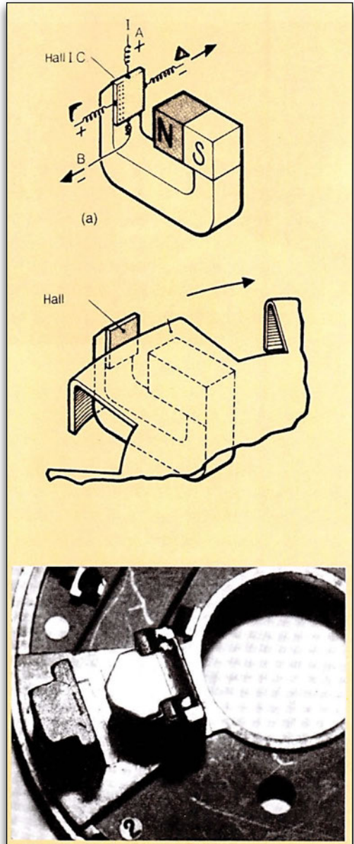
Εικόνα 3.2.3 Αισθητήρας Hall
