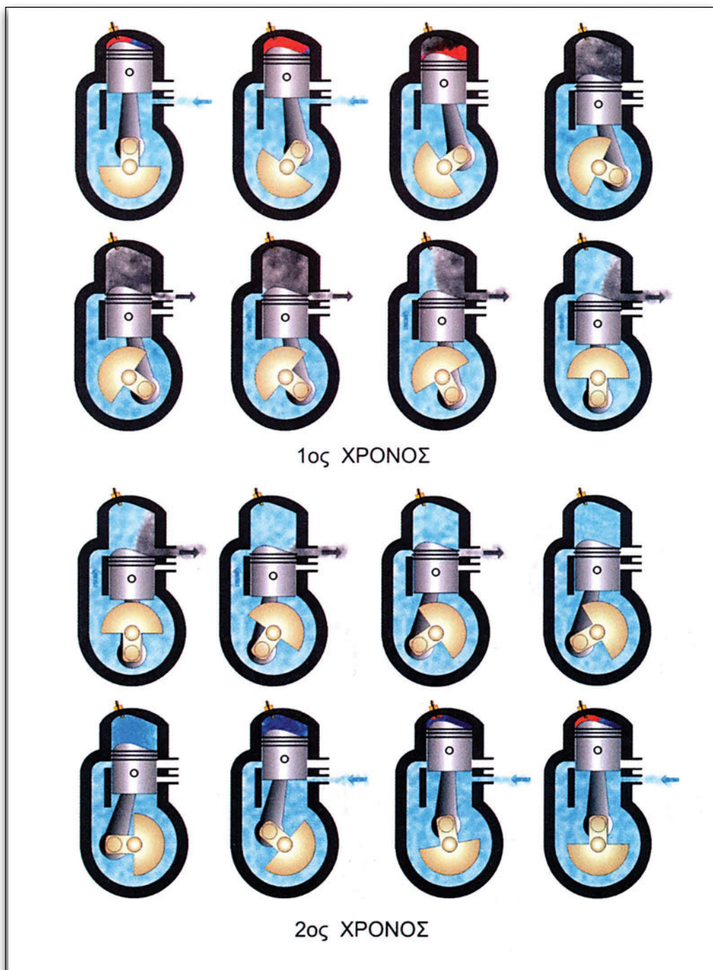
Εικόνα 1.2.12 Χρόνοι λειτουργίας και εξέλιξη των φάσεων δίχρονου βενζινοκινητήρα
