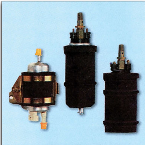
Εικόνα 3.1.8 Αντλίες γραμμής
