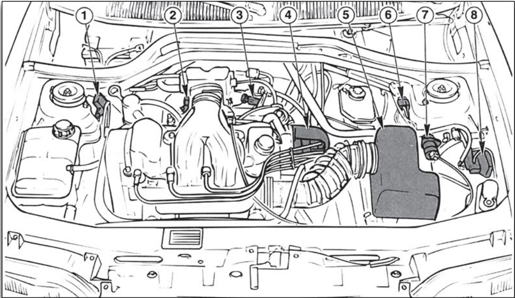
Εικόνα 3.3.10 Κινητήρας με σύστημα EFI
