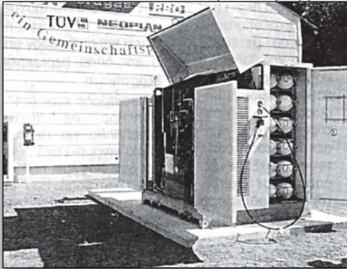
Εικόνα 7.1.11 Σταθμός πλήρωσης φυσικού αερίου στη Γερμανία
