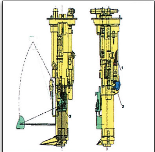
Εικόνα 3.1.9 Εμβαπτιζόμενη αντλία με φλοτέρ
