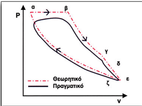
Εικόνα 1.2.14 Θεωρητικό και πραγματικό διάγραμμα δίχρονου πετρελαιοκινητήρα
