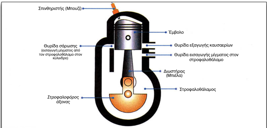
Εικόνα 1.2.9 2χρονος βενζινοκινητήρας
