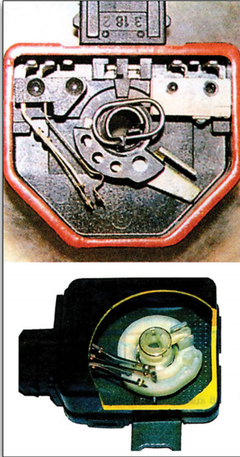
Εικόνα 3.1.36 Διακόπτης πεταλούδας
