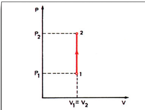
Εικόνα 1.1.3 Ισόχωρη μεταβολή
