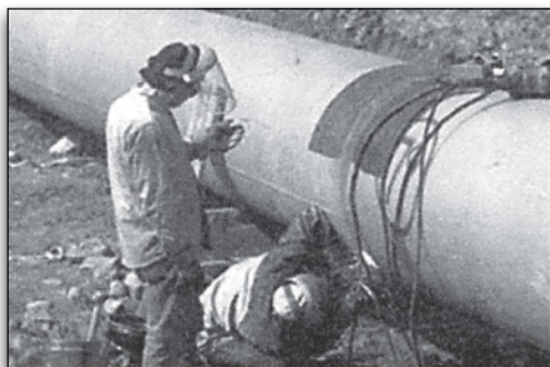
Εικόνα 7.1.8 Κατασκευή αγωγού μεταφοράς φυσικού αερίου στη Σιβηρία
