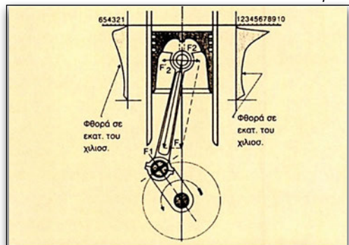
Εικόνα 2.2.1 Δυνάμεις στο έμβολο ενός κυλίνδρου
