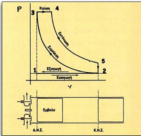
Εικόνα 1.2.5β Θεωρητικό διάγραμμα λειτουργίας τετράχρονου πετρελαιοκινητήρα
