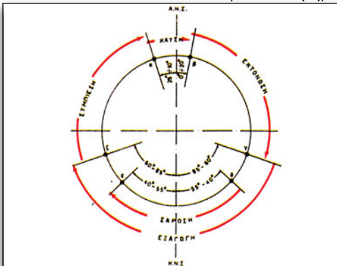
Εικόνα 1.2.15 Κυκλικό διάγραμμα δίχρονου πετρελαιοκινητήρα
