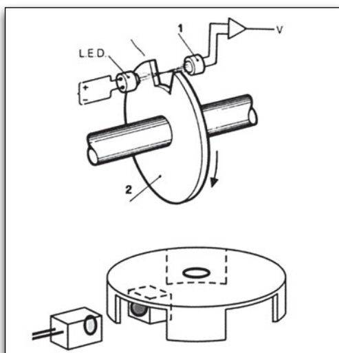
Εικόνα 3.2.5 οπτικός αισθητήρας
