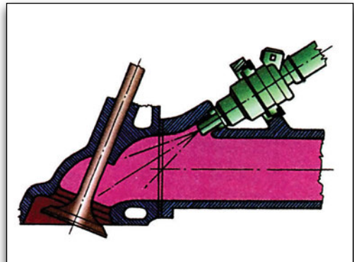
Εικόνα 3.1.1 Μπεκ βενζίνης
