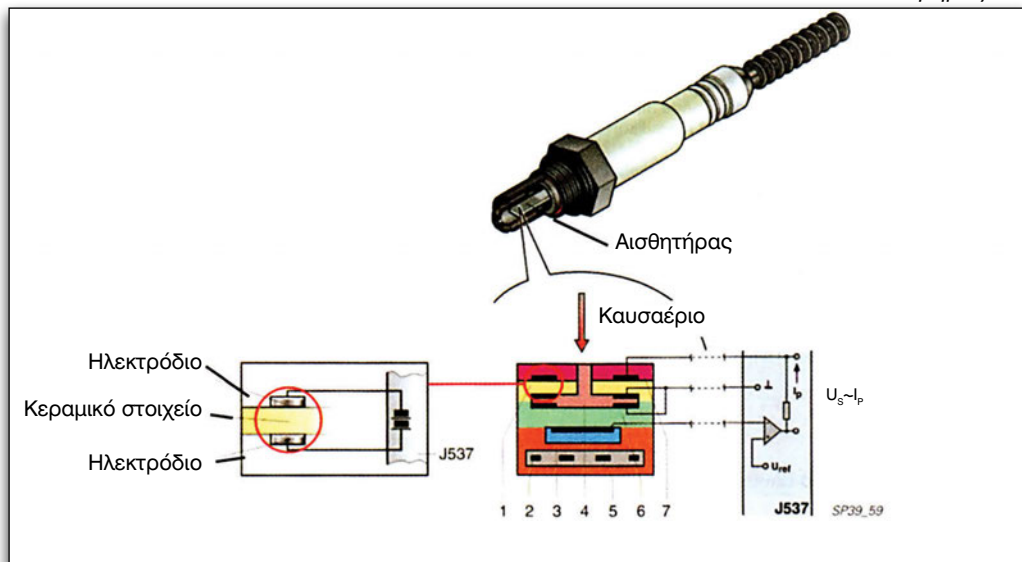
Εικόνα 4.2.13 Αισθητήρας “λ”.
