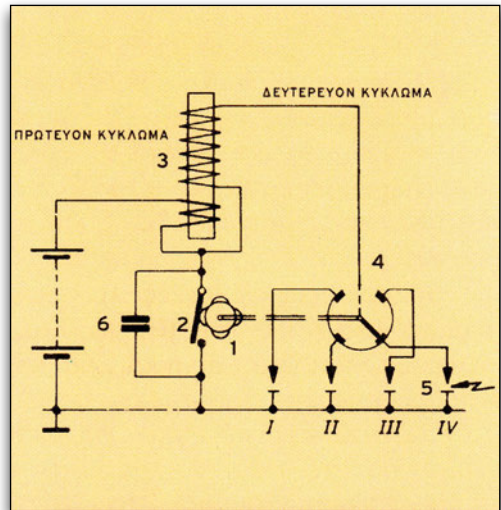
Εικόνα 3.2.1 Ηλεκτρικό κύκλωμα ανάφλεξης με πλατίνες
