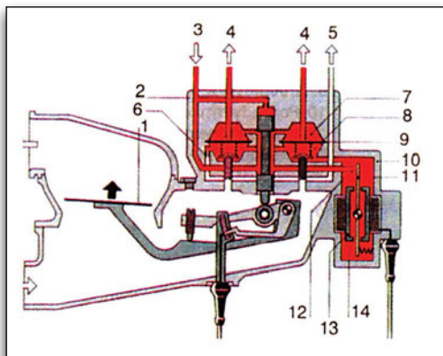
Εικόνα 3.1.49. Διανομέας με ηλεκτροϋδραυλικό ρυθμιστή
