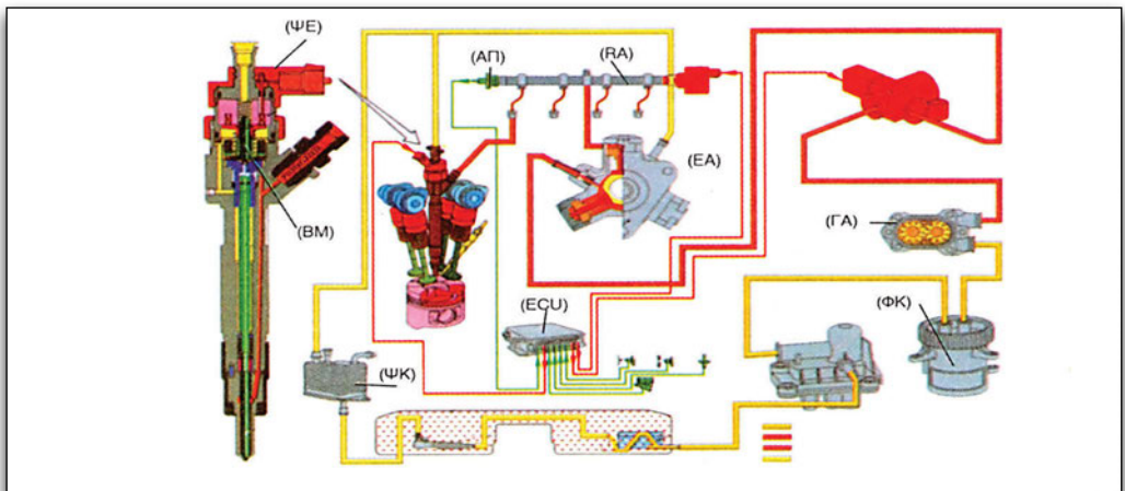
Εικόνα 6.1.8 Σύστημα Common-Rail.
