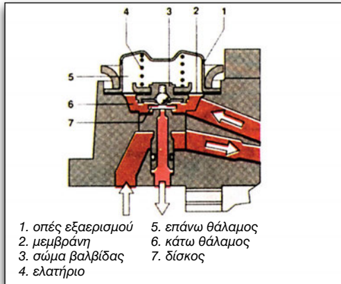
Εικόνα 3.1.23 Μπεκ μονού ψεκασμού με το ρυθμιστή πίεσης
