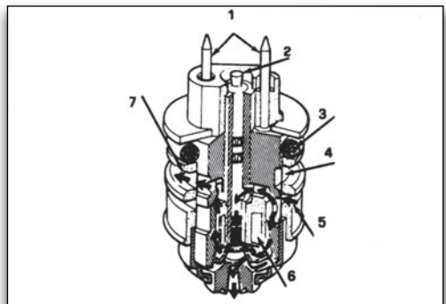
Εικόνα 3.1.18 Μπεκ κεντρικού ψεκασμού 6 οπών γωνίας ψεκασμού 45° με σφαιρική έδραση
