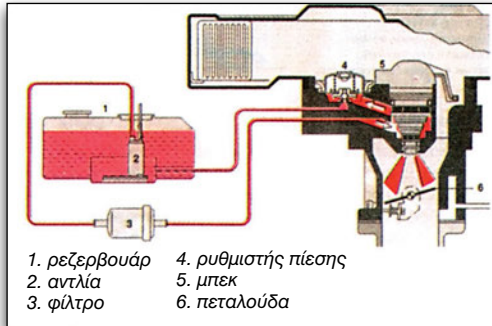
Εικόνα 3.1.22 Ρυθμιστής πίεσης
