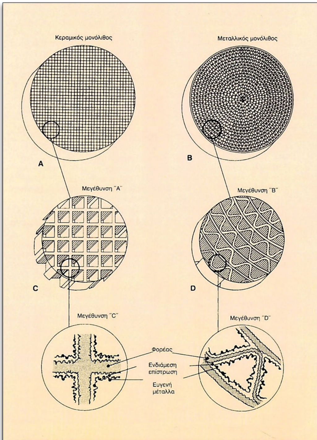
Εικόνα 4.2.9 Χαρακτηριστικά καταλυτικών μετατροπέων
