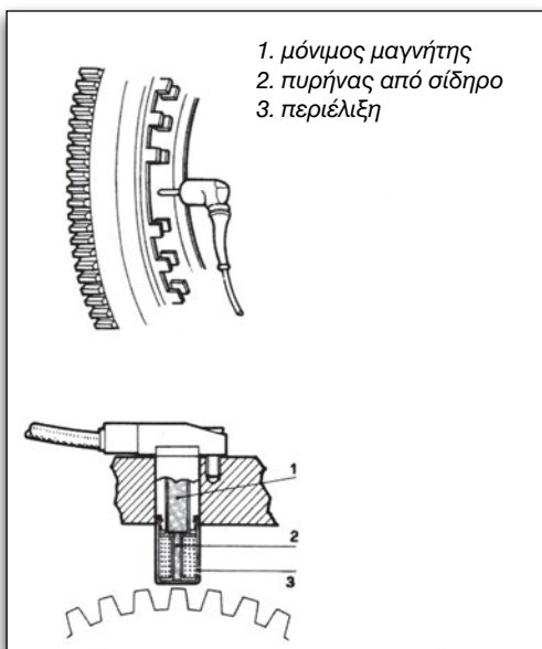
Εικόνα 3.2.14 Αισθητήρας στροφών και γωνίας στροφαλοφόρου (κάτω)
