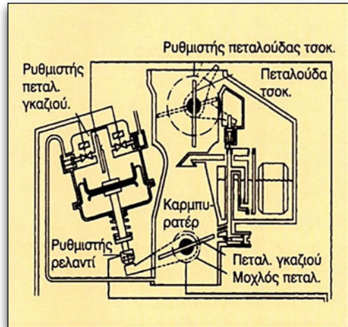
Εικόνα 4.2.11 Ηλεκτρικά ρυθμιζόμενο καρμπυρατέρ
