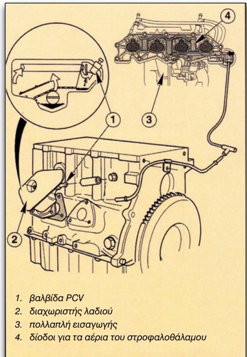
Εικόνα 4.1.13 Εξαερισμός στροφαλοθάλαμου
