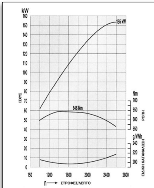
Εικόνα 8.1.4 Διάγραμμα ισχύος - ροπής και ειδικής κατανάλωσης καυσίμου κινητήρα Η χαμηλότερη ειδική κατανάλωση
