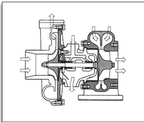
Εικόνα 2.5.4 Στροβιλοσυμπίεστής
