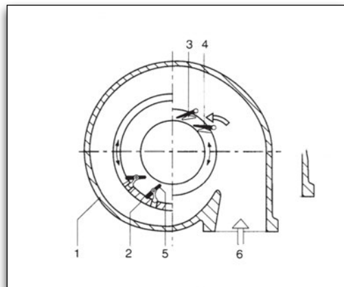
Εικόνα 2.5.9 Στροβιλοσυμπιεστές με ρυθμιζόμενα πτερύγια
