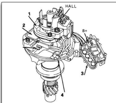
Εικόνα 3.2.6 Ανάφλεξη HEI
