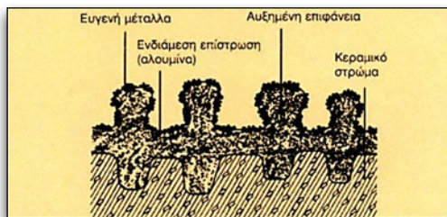
Εικόνα 4.2.8 Επίστρωση αλουμίνιας.
