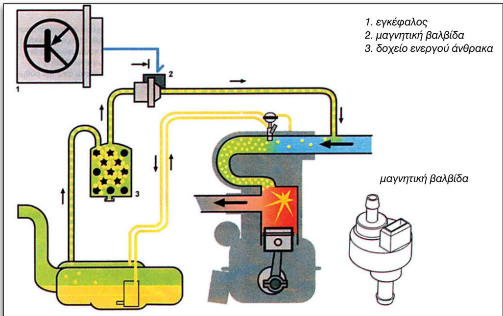
Εικόνα 4.1.4 Εξαερισμός ρεζερβουάρ
