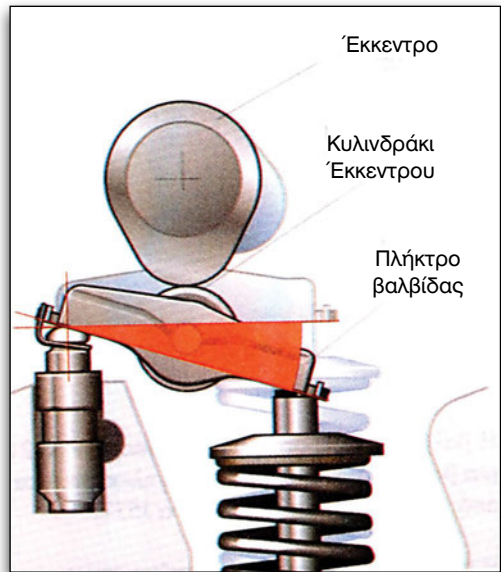
Εικόνα 2.3.4 Εκκεντροφόρος επικεφαλής, επιδρά στη βαλβίδα μέσω ζυγώνθρου
