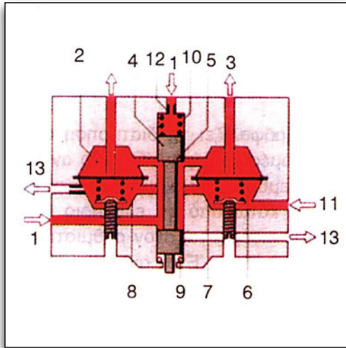
Εικόνα 3.1.48 Διανομέας καυσίμου
