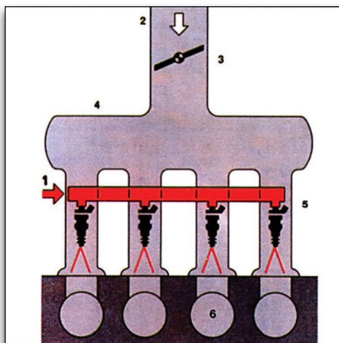
1. καύσιμο 4. πολλαπλή εισαγωγής 2. αέρας 5. μπεκ 3. πεταλούδα 6. κινητήρας
