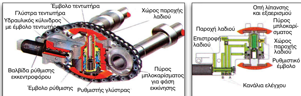
Εικόνα 2.3.7 Ρυθμιστής εκκεντροφόρου
