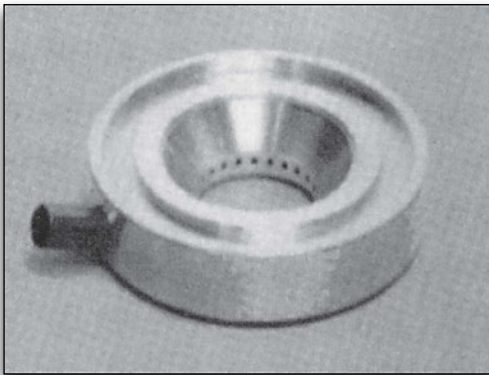
Εικόνα 7.2.6 Δακτύλιος ανάμειξης υγραερίου - αέρα (αναμείκτης)
