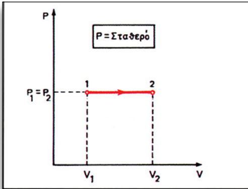
Εικόνα 1.1.2. Ισοβαρής μεταβολή
