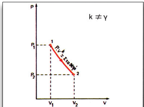
Εικόνα 1.1.5 Πολυτροπική μεταβολή
