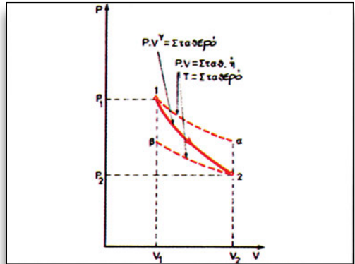
Εικόνα 1.1.4 Αδιαβατική μεταβολή
