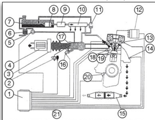
Εικόνα 3.3.9 Συνδεσμολογία Multec
