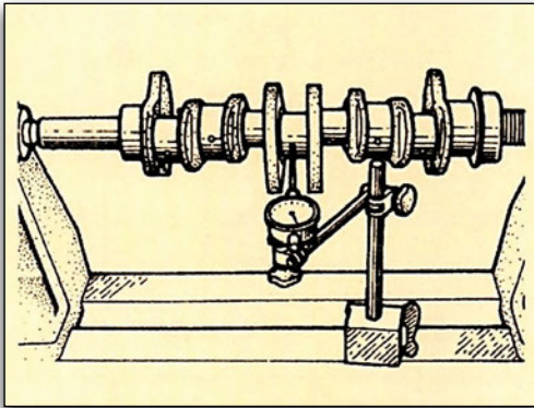
Εικόνα 2.2.8 Μέτρηση στρέβλωσης στροφοφόρου άξονα
